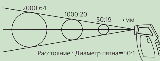
АКИП-9306, АКИП-9307
